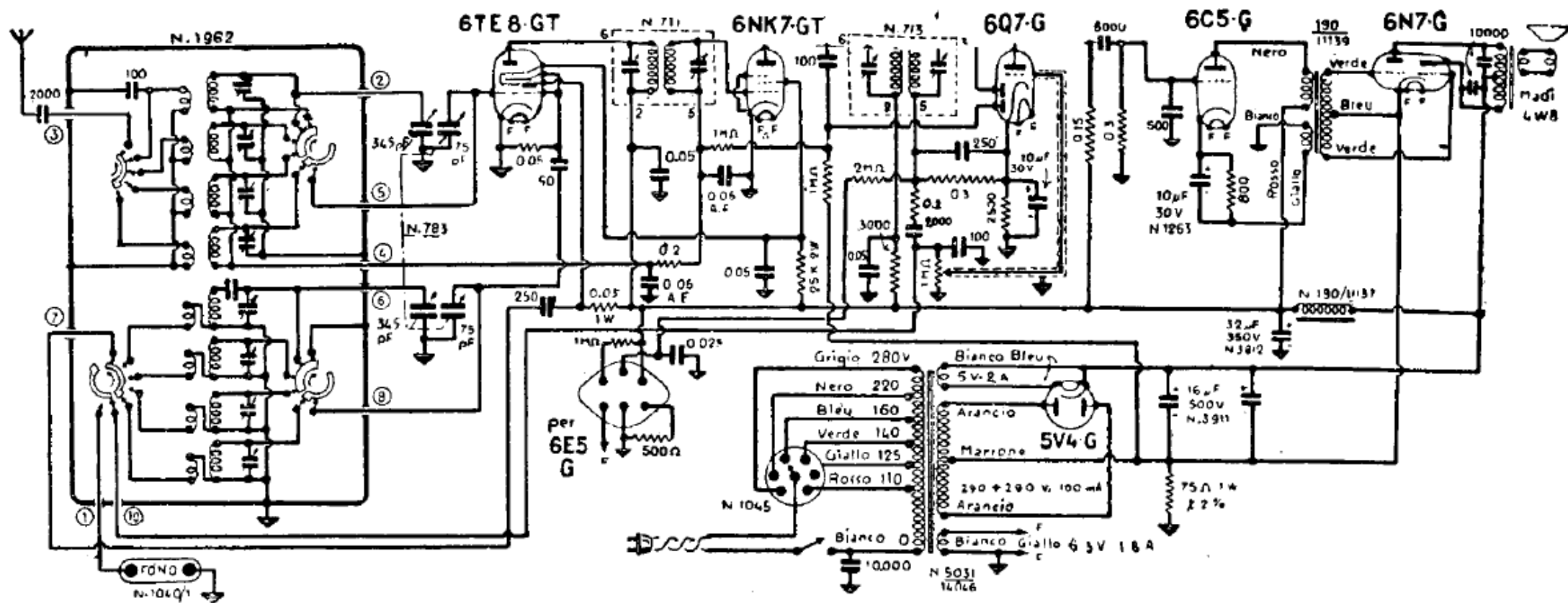
GELOSO. — Mod. G. 77 R. — AF e MF come G. 75 R. — Media frequenza: 467 kHz. — Potenza: 10 W. — Produzione 1946-47.
